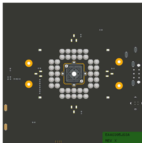
EAA0395J03A Rev D – AMG mit 2 Kameras
